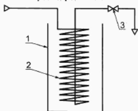
1 — сосуд для охлаждающей смеси; 2 — змеевик; 3 — игольчатый вентиль
