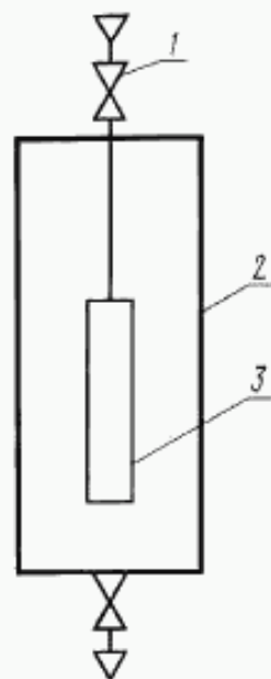
1 — игольчатый вентиль; 2 — корпус; 3 — медная пластинка
