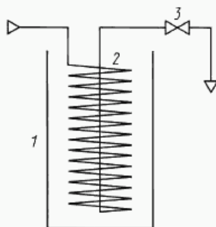
Устройство для охлаждения сжиженного углеводородного газа
